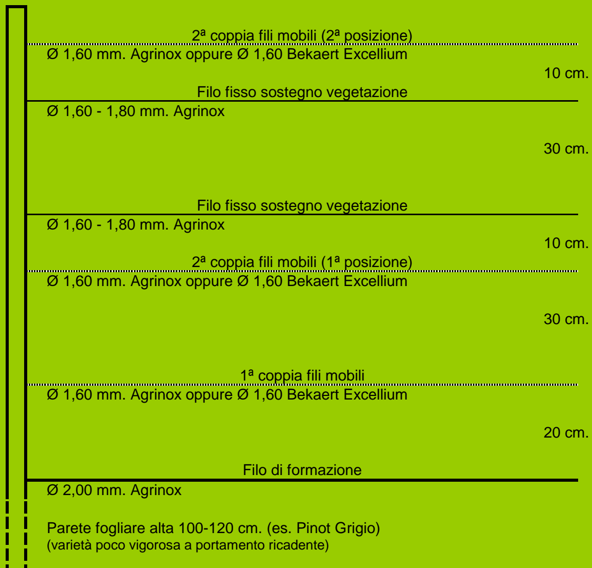
GRAFICO B: es. soluzione con 2 coppie di fili mobili
